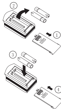
Σκαρήφμα αντικατάστασης μπαταριών
