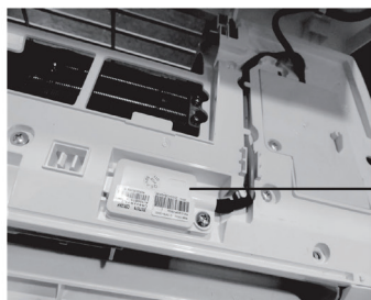
Modulul Wi-Fi
