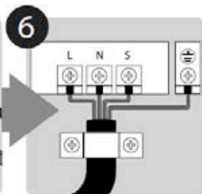
6 Conectați cablurile (pagina 17)
