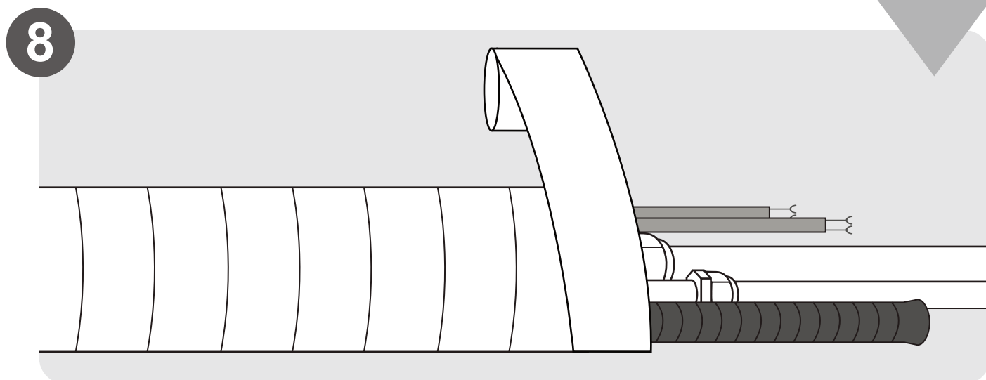
8 Înveliți conductele și cablurile (condiție neaplicabila în anumite zone din Statele Unite ale Americii). (pagina 19)
