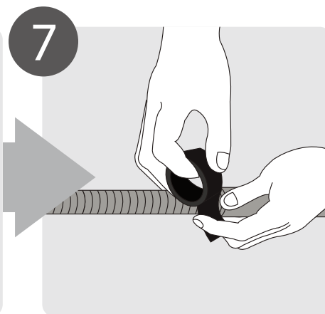
7 Προετοιμάστε τον αγωγό αποστράγγισης (Σελίδα 16)
