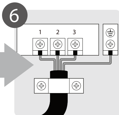
6 Συνδέστε τις καλωδιώσεις (Σελίδα 17)
