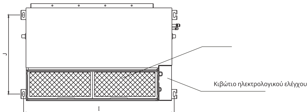
Κατερχόμενο άνοιγμα εξαερισμού και τοποθετημένο άγκιστρο
