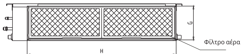
Διαστάσεις εισόδου αέρα
